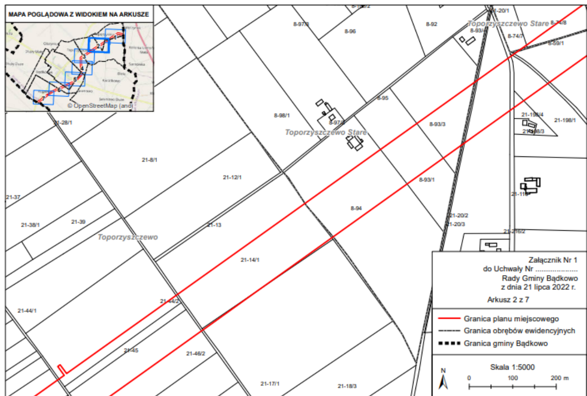
Rysunek 5 Projekt miejscowego planu zagospodarowania przestrzennego dla dwutorowej napowietrznej linii elektroenergetycznej arkusz 2 z 7
