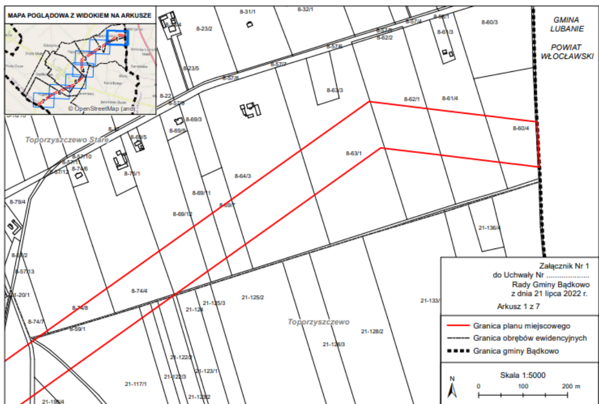
Rysunek 4 Projekt miejscowego planu zagospodarowania przestrzennego dla dwutorowej napowietrznej linii elektroenergetycznej arkusz 1 z 7
