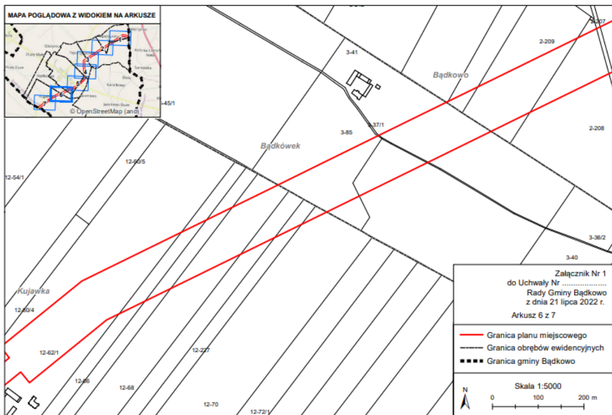
Rysunek 9 Projekt miejscowego planu zagospodarowania przestrzennego dla dwutorowej napowietrznej linii elektroenergetycznej arkusz 6 z 7
