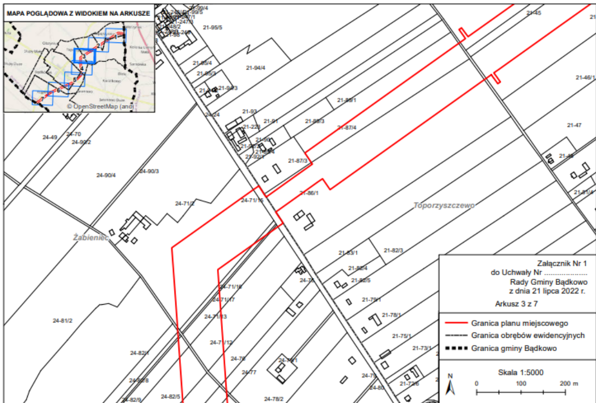
Rysunek 6 Projekt miejscowego planu zagospodarowania przestrzennego dla dwutorowej napowietrznej linii elektroenergetycznej arkusz 3 z 7
